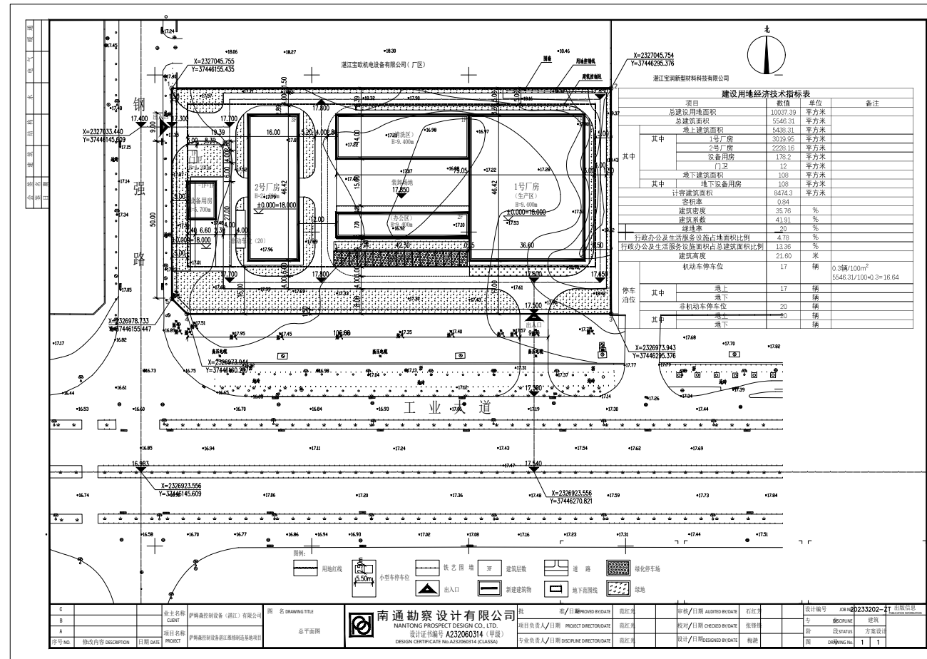
总平面图
