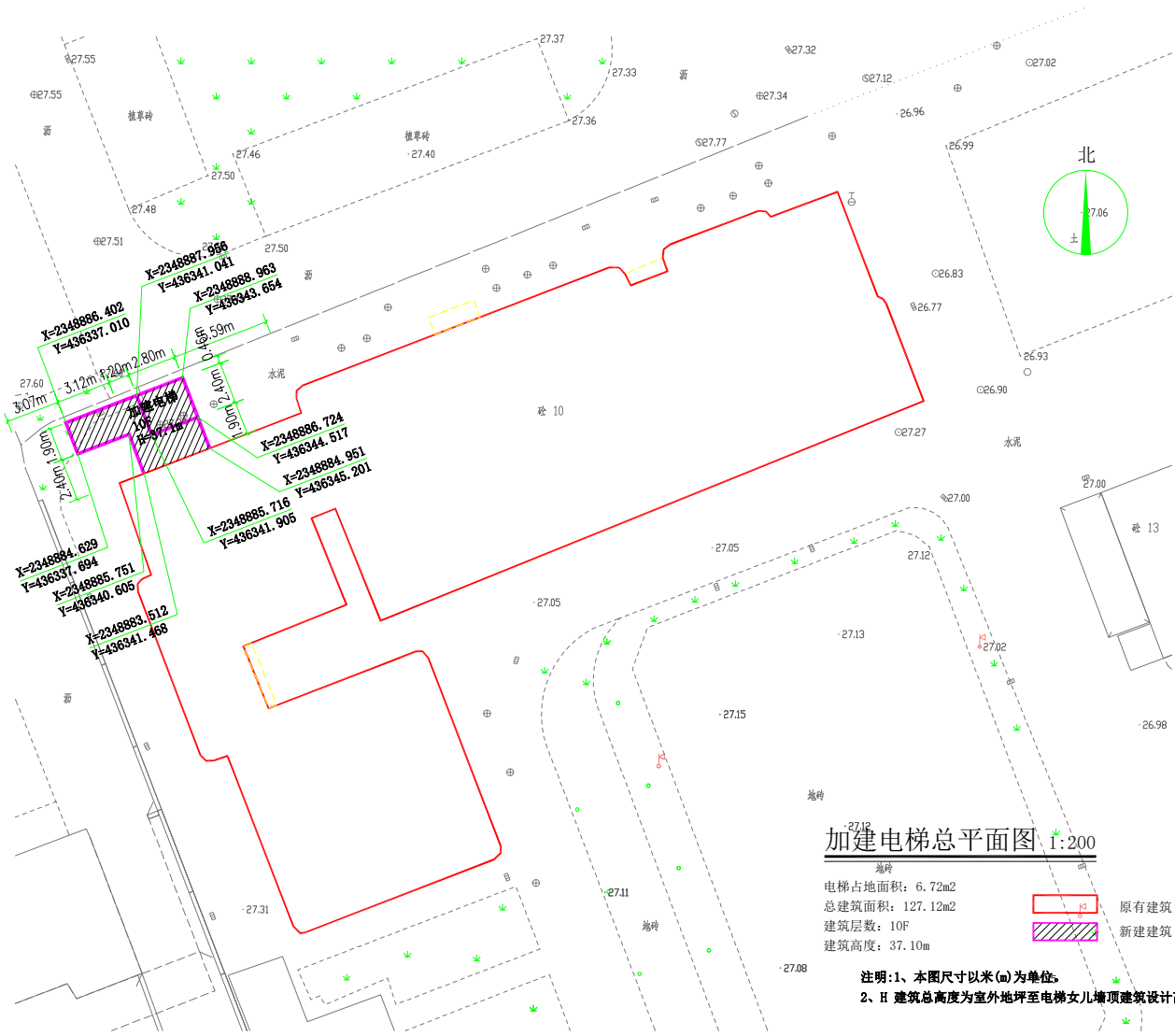
总平面图
