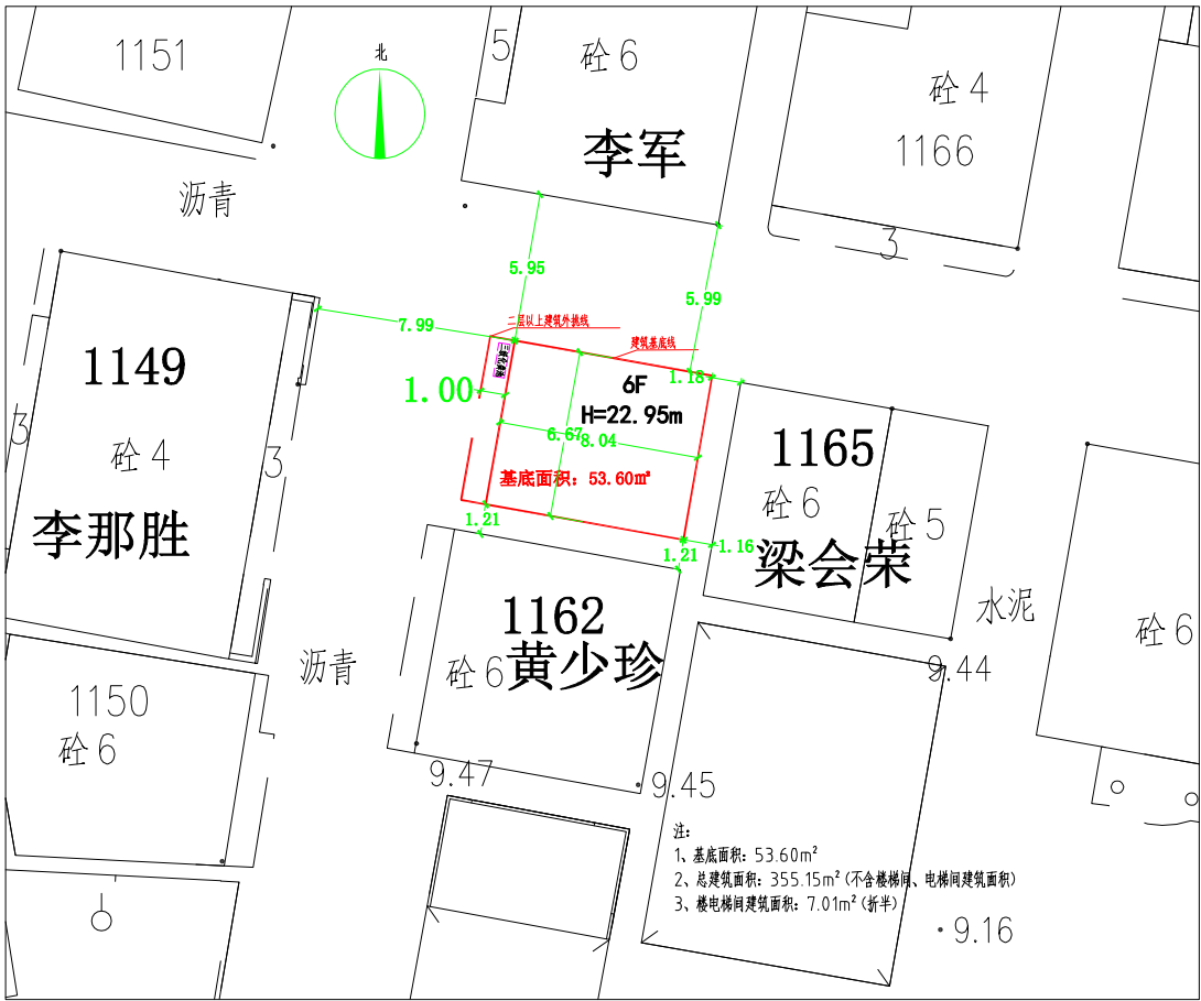
四至总平面图
