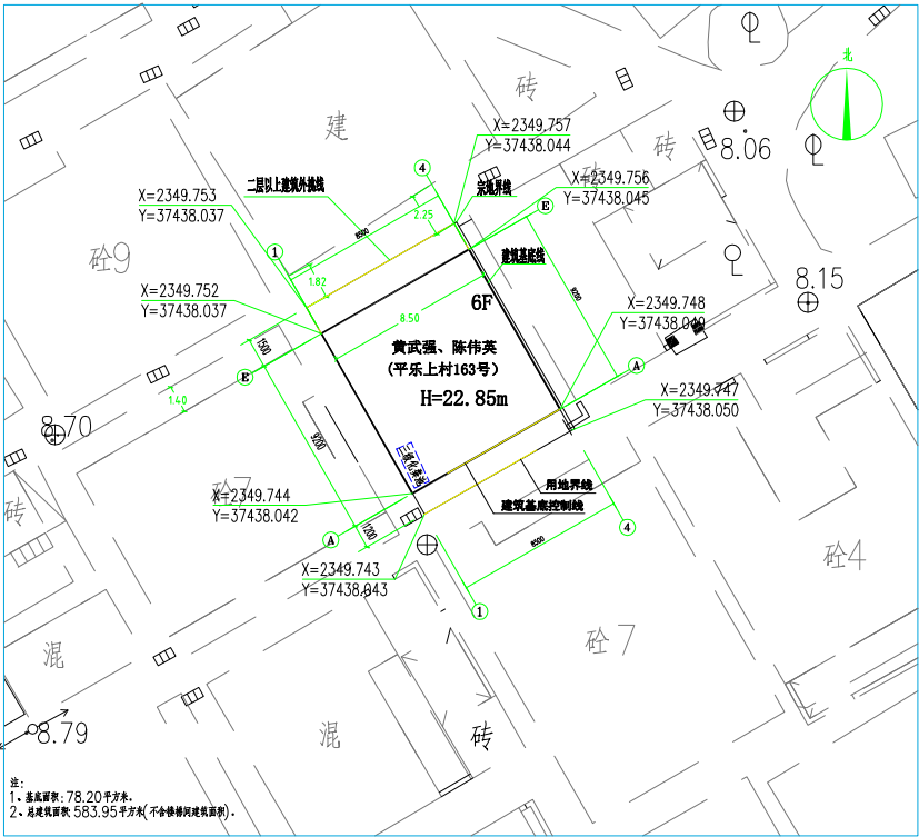
四至总平面图
