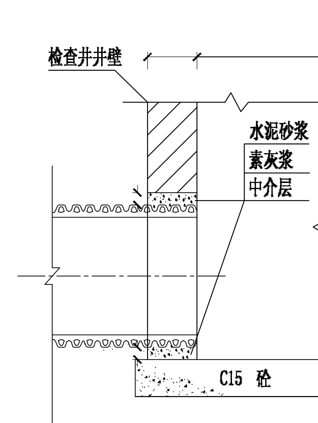
管道与检查井接口示意图
