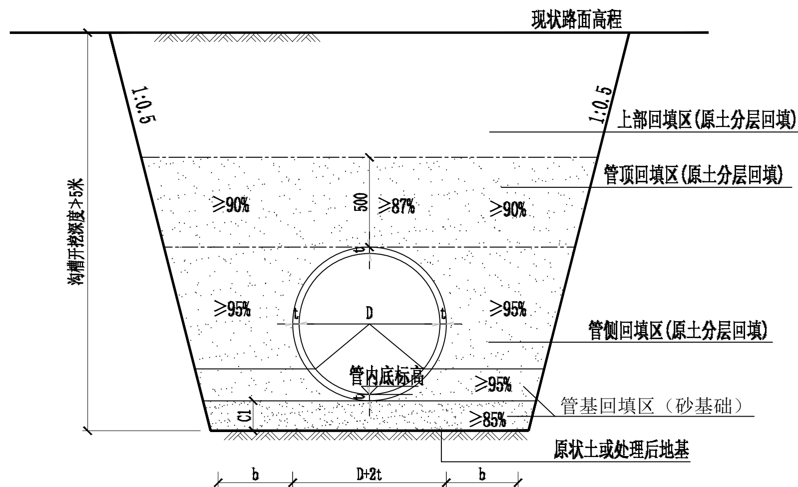
塑料管挖基断面图
