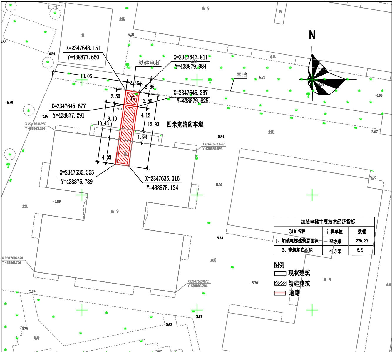
总平面图
