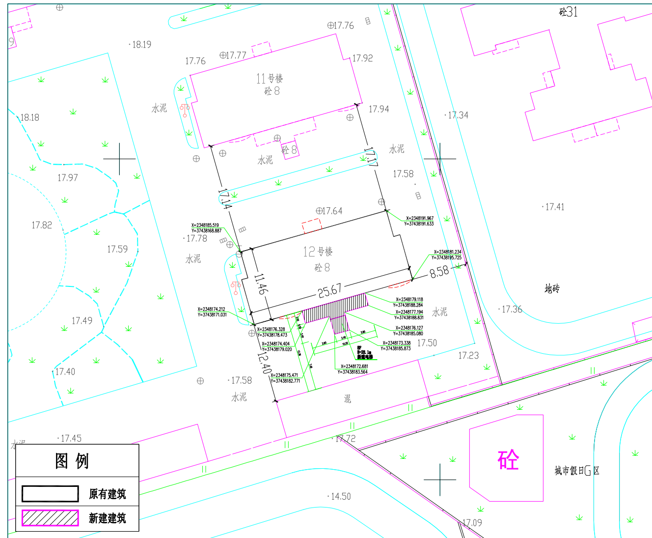
总平面图
