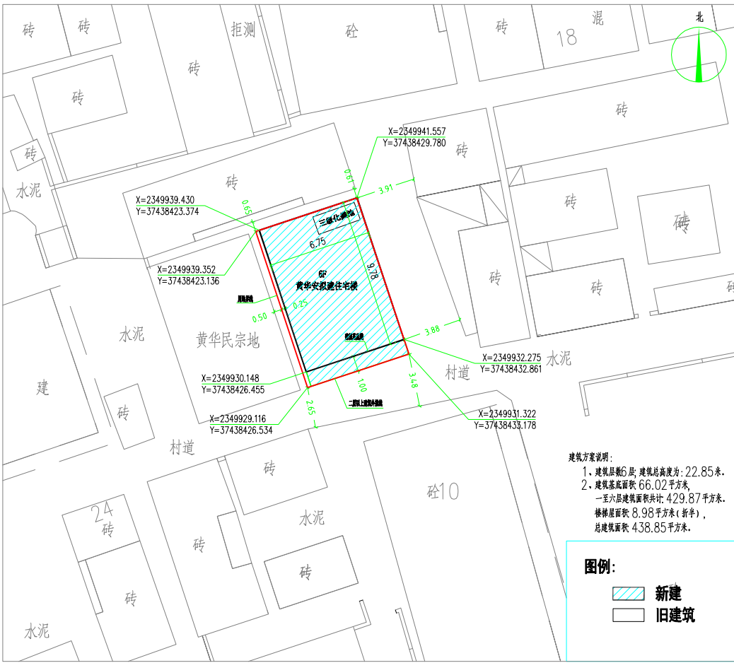
四至总平面图
