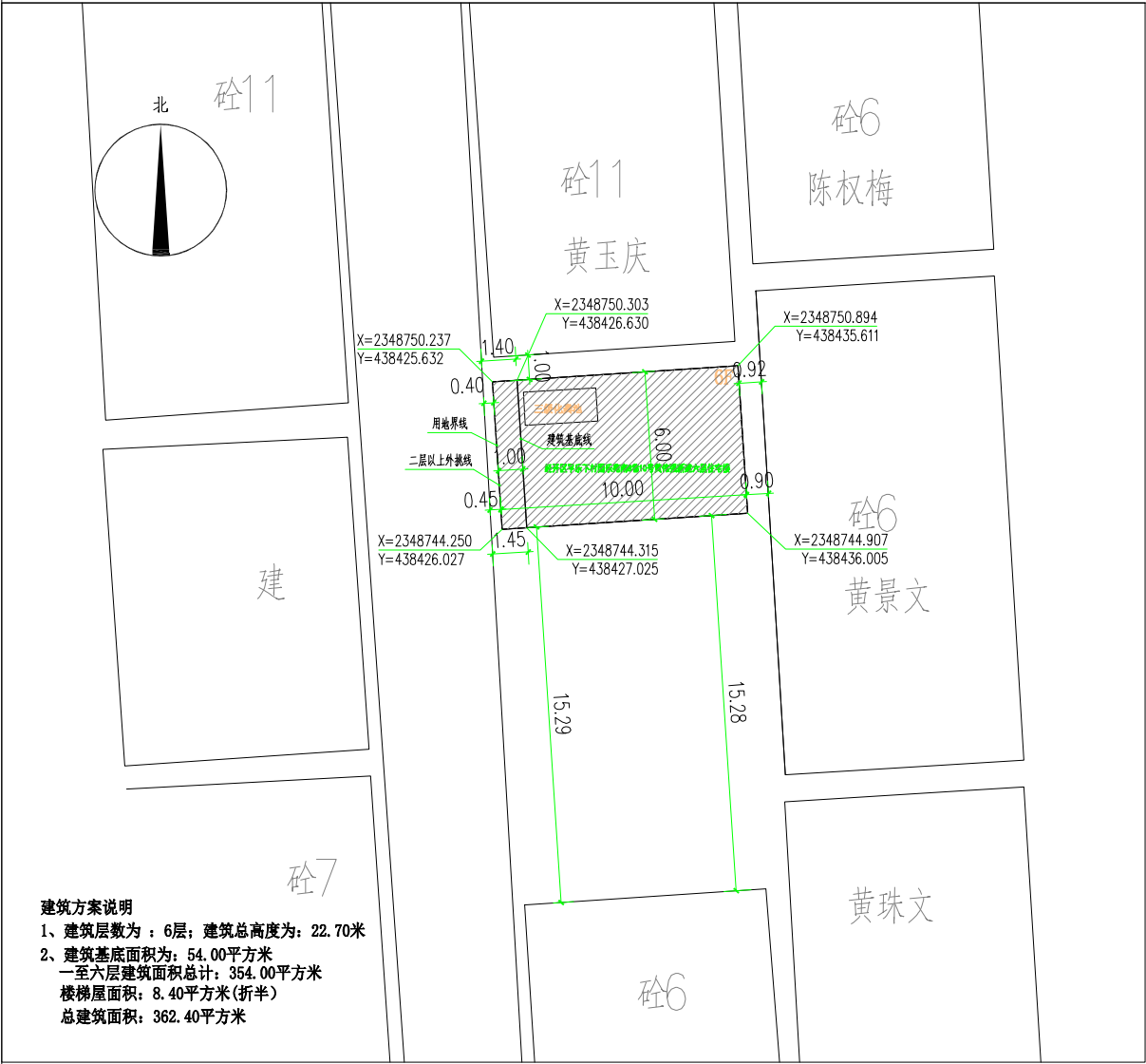
四至总平面图
