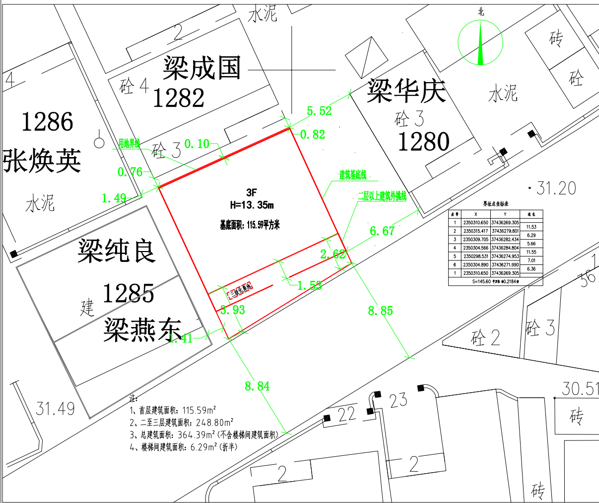
四至总平面图
