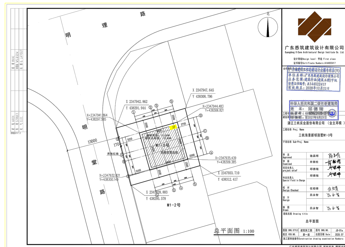
总平面图
