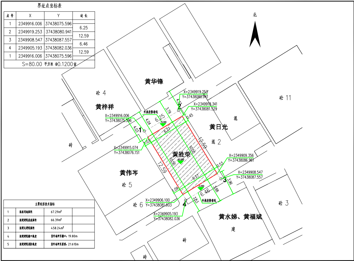
四至总平面图
