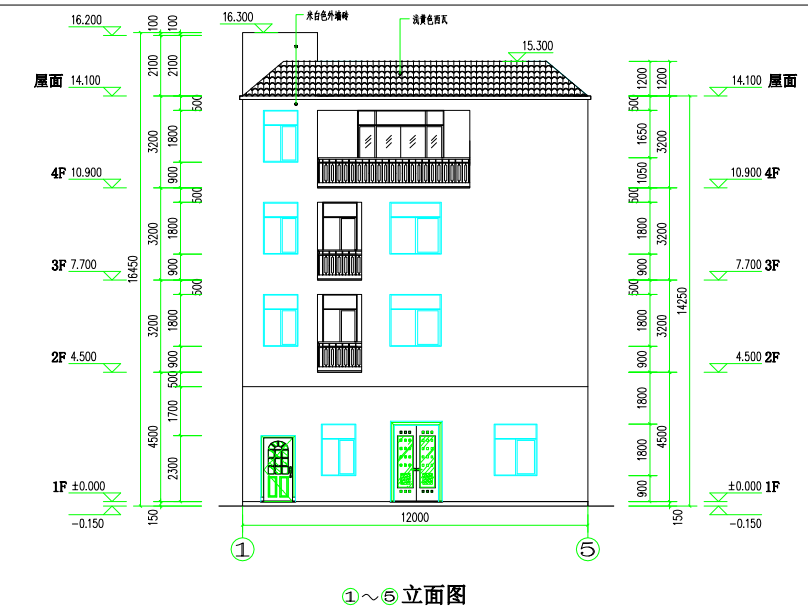
①~⑤ 立面图
