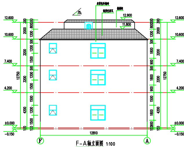
F-A轴立面图 1:100
