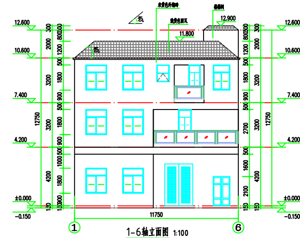
1-6轴立面图 1:100
