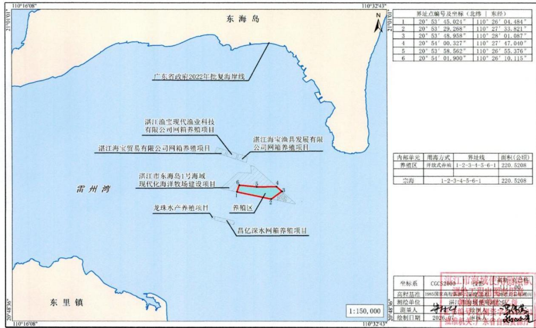
广东省深海牧渔科技有限公司现代化海洋牧场建设项目宗海界址图
