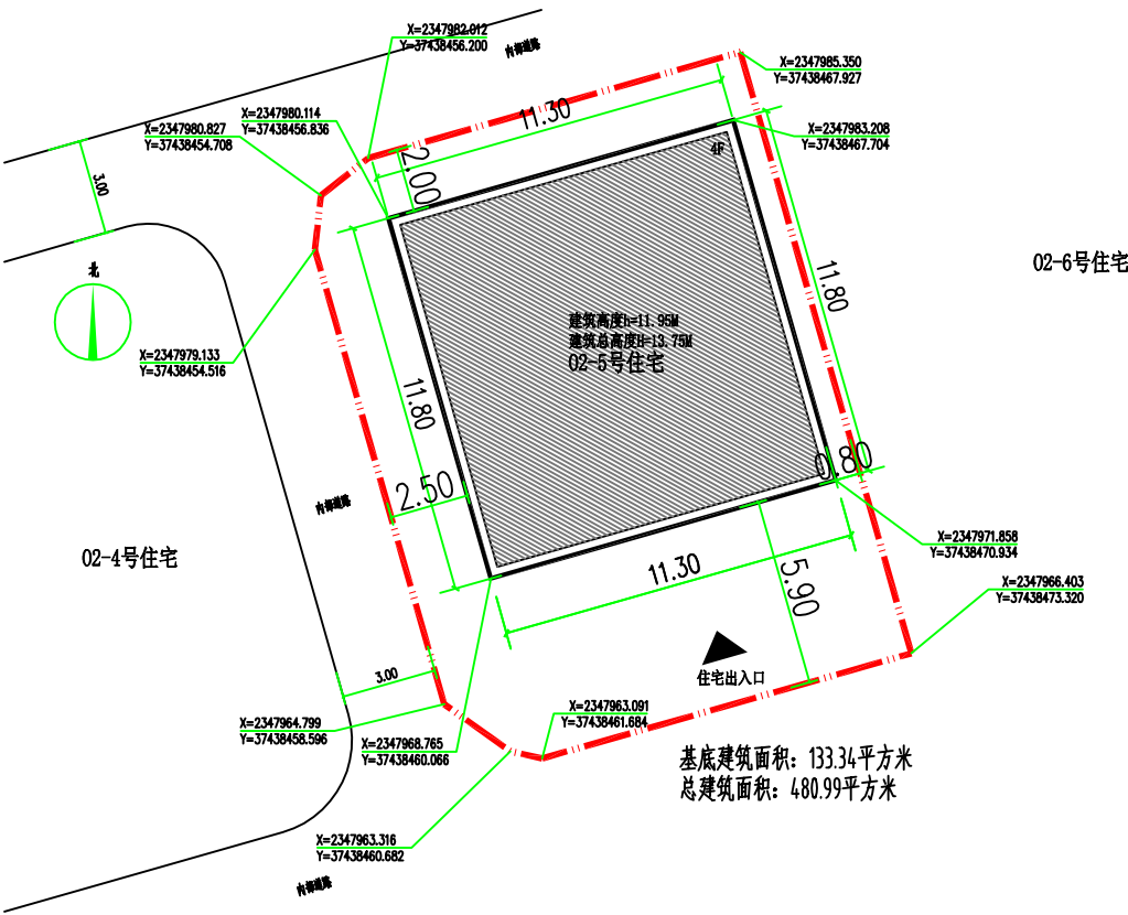
总平面图
