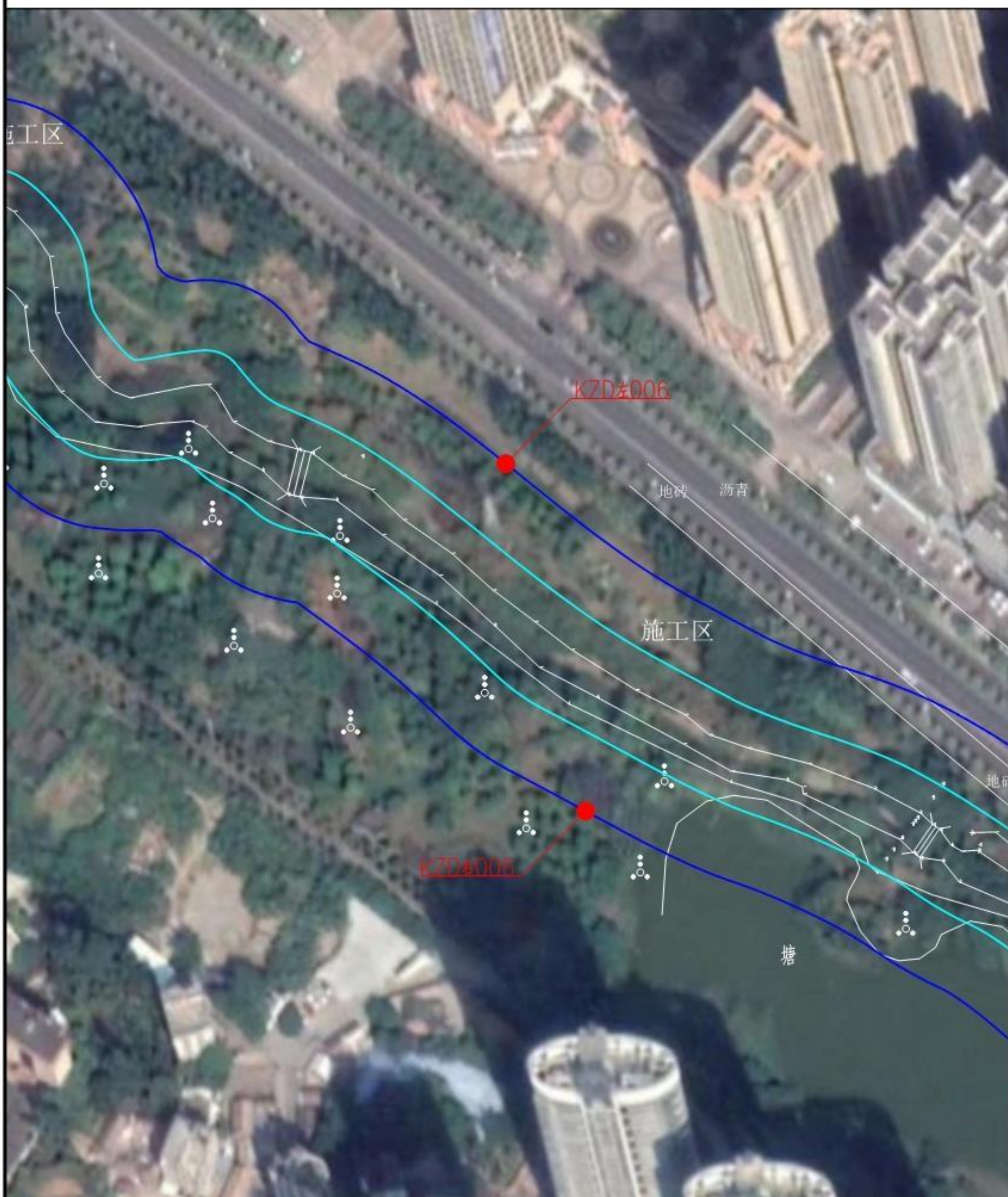
绿塘渠湛江开发区段河道管理范围线平面布置图(7/14)
