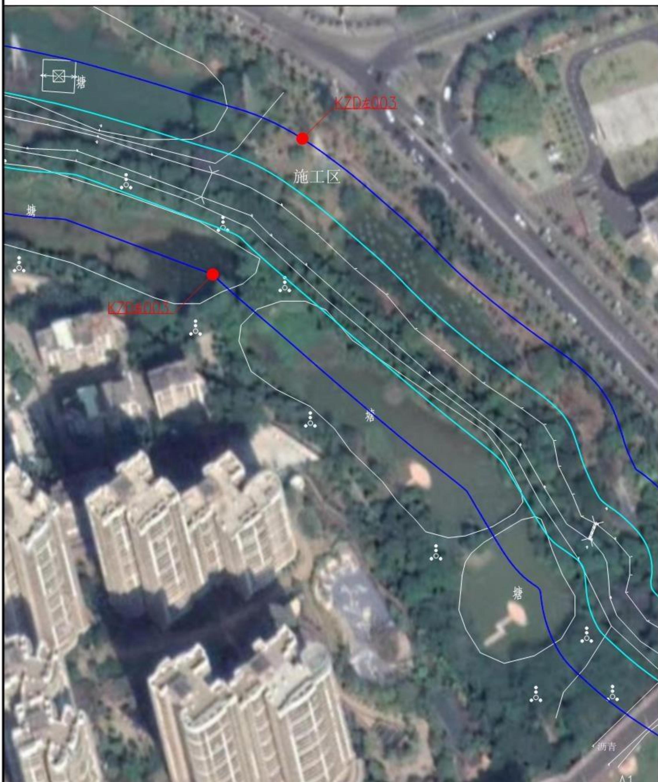
绿塘渠湛江开发区段河道管理范围线平面布置图(3/14)
