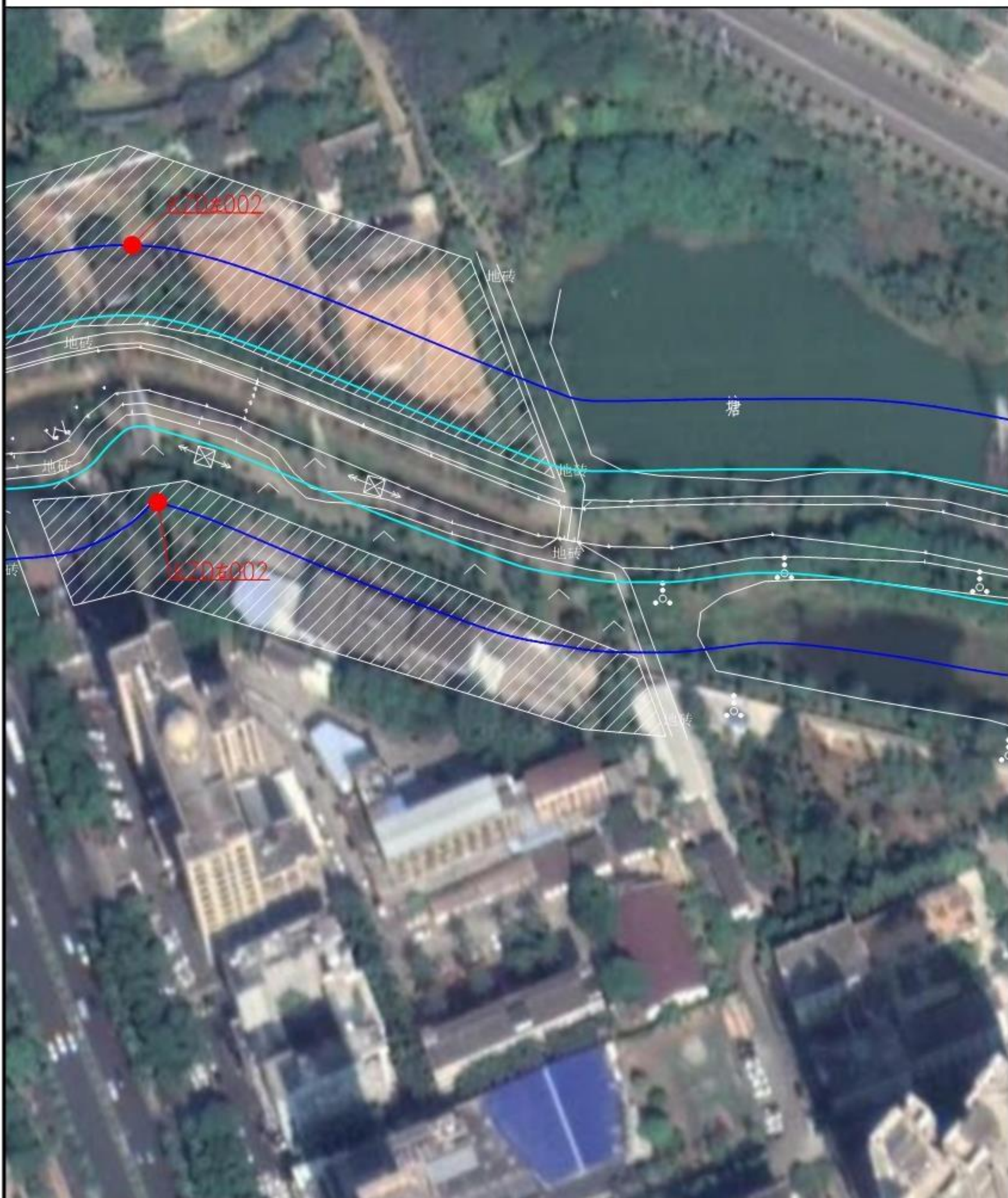
绿塘渠湛江开发区段河道管理范围线平面布置图(2/14)
