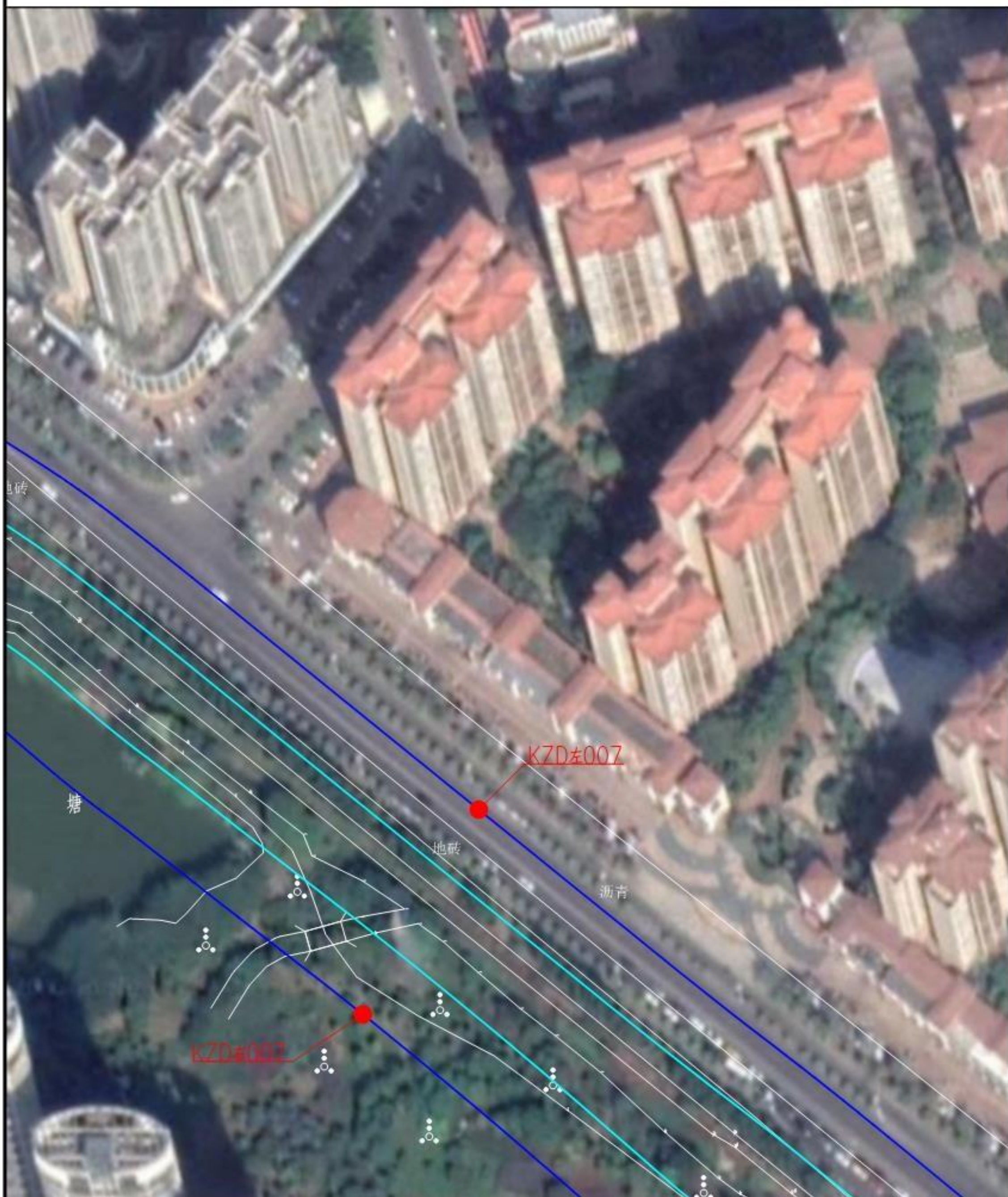
绿塘渠湛江开发区段河道管理范围线平面布置图(8/14)
