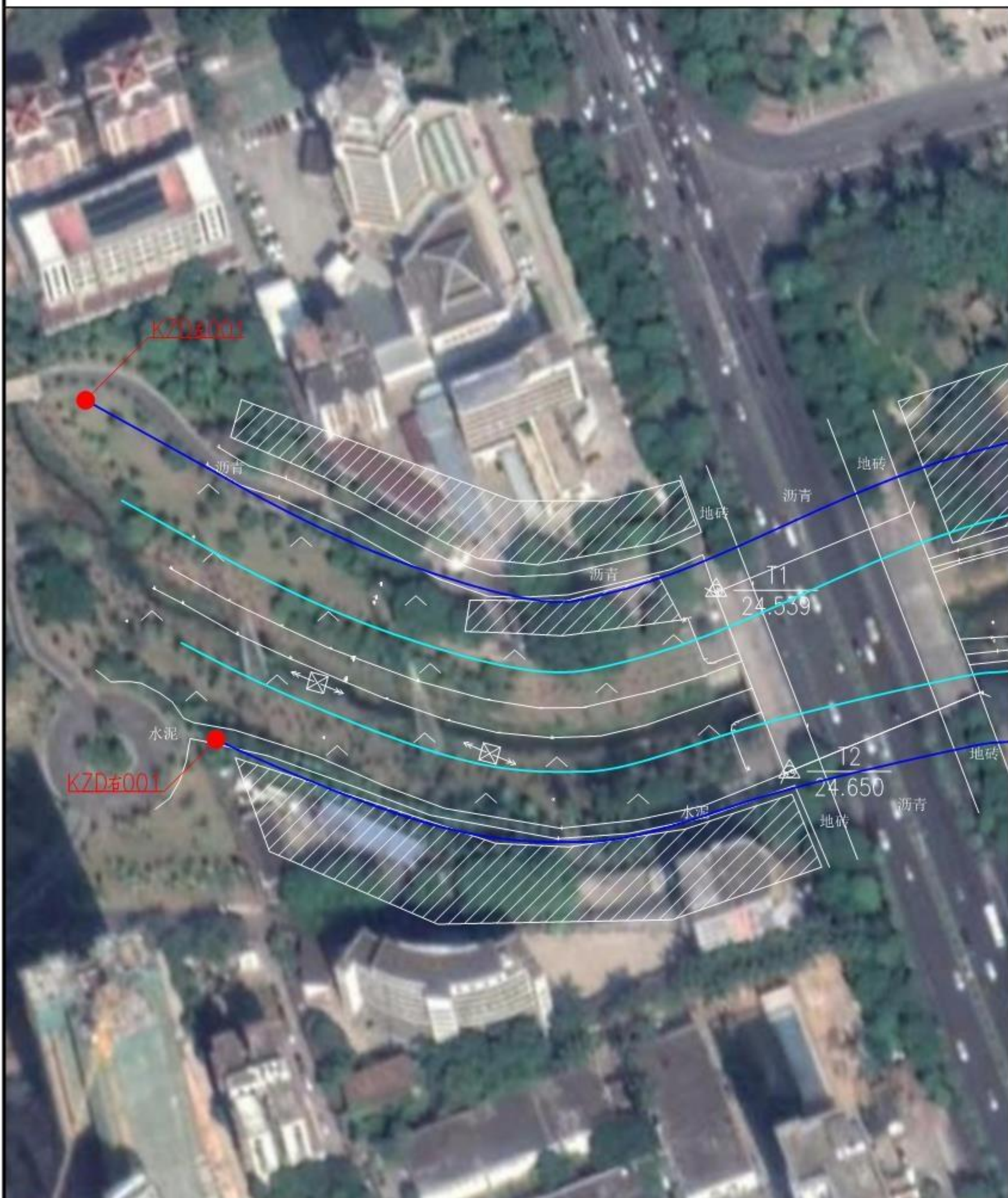
绿塘渠湛江开发区段河道管理范围线平面布置图(1/14)
