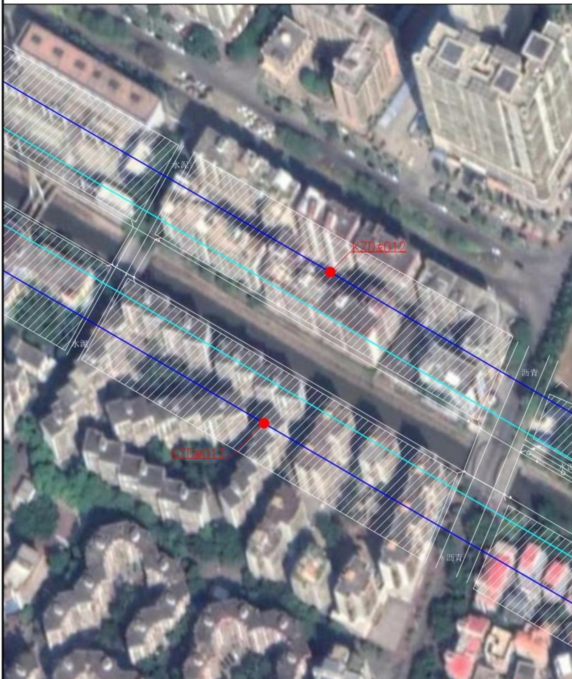
绿塘渠湛江开发区段河道管理范围线平面布置图(13/14)
