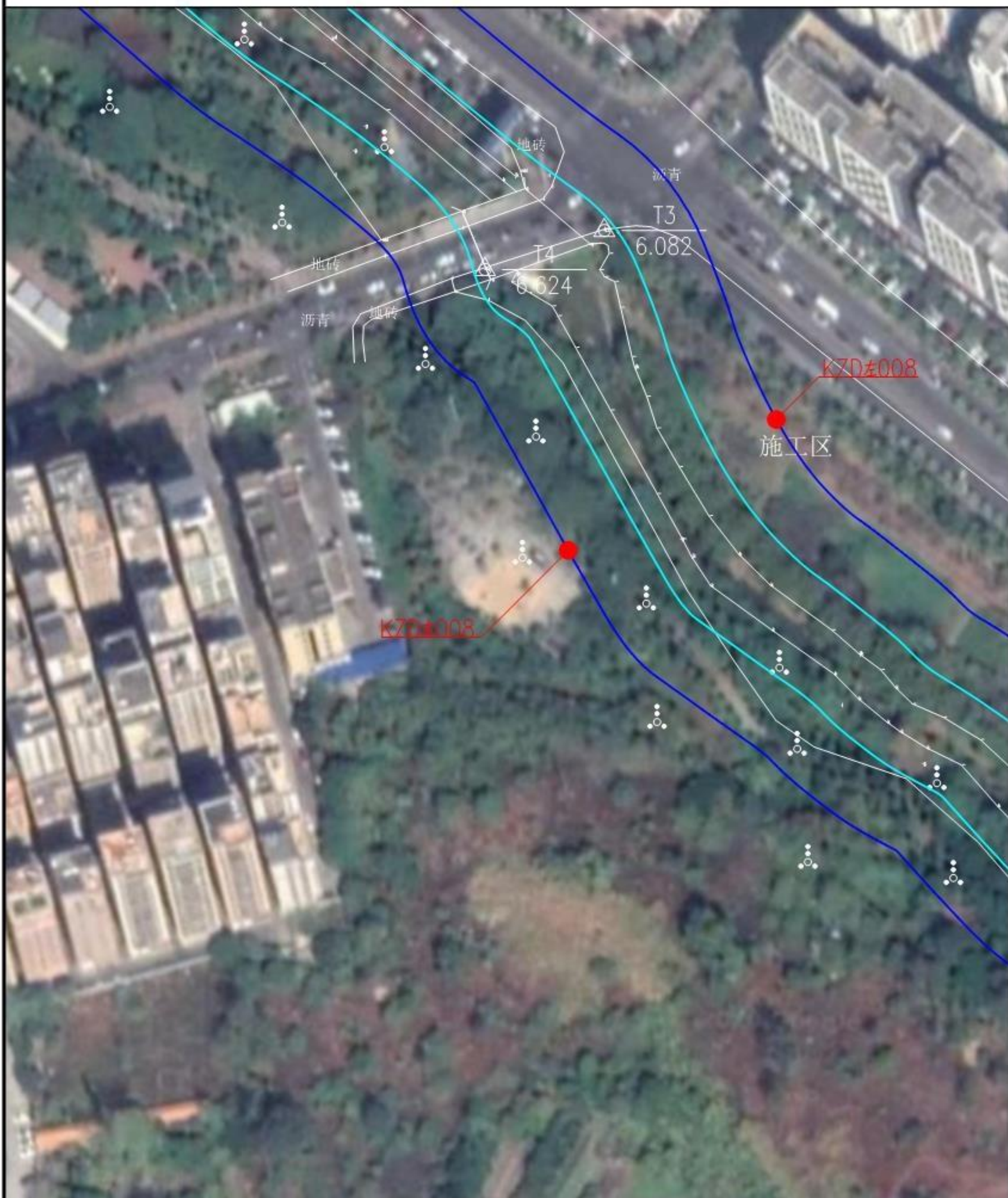
绿塘渠湛江开发区段河道管理范围线平面布置图(9/14)
