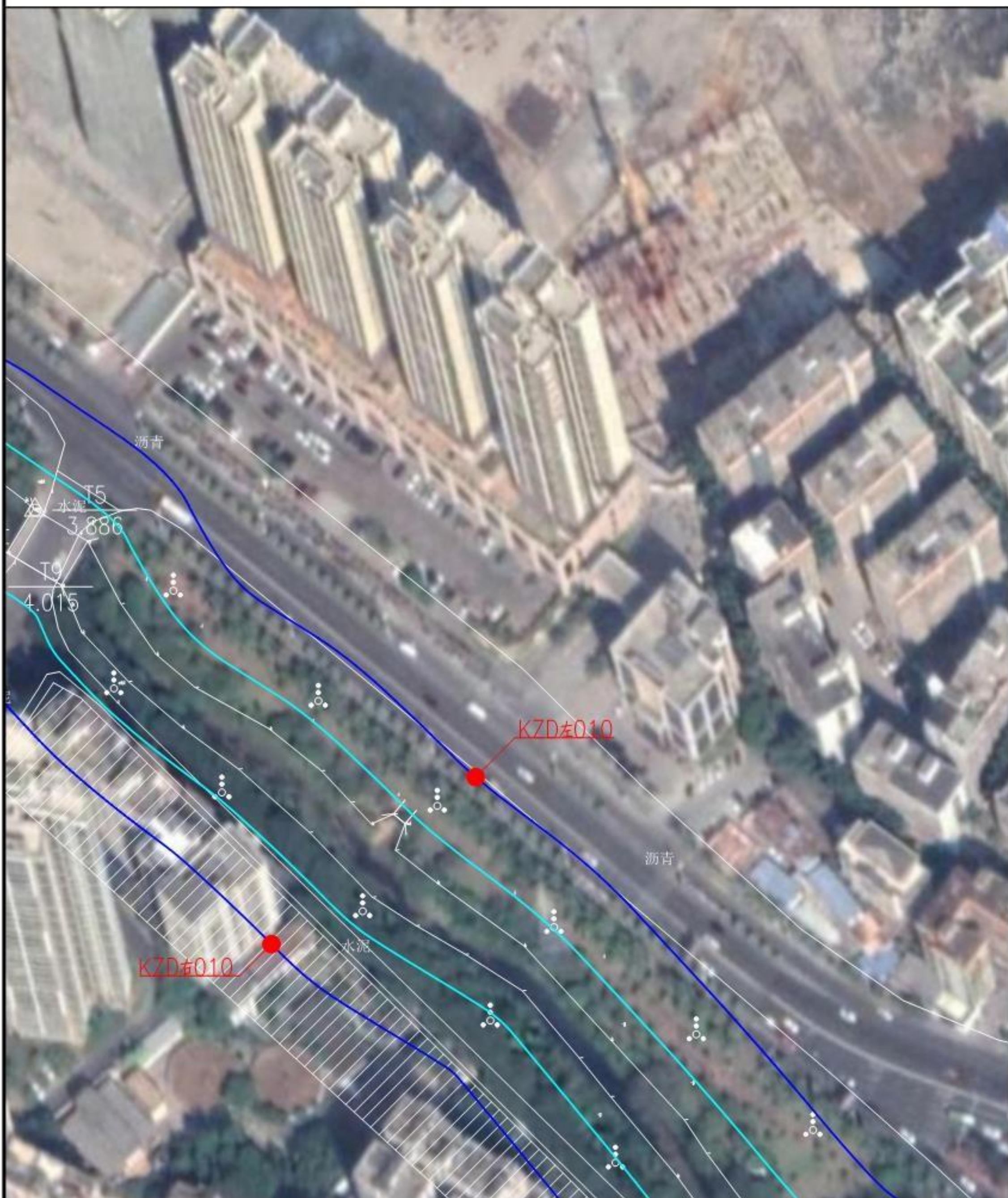
绿塘渠湛江开发区段河道管理范围线平面布置图(11/14)
