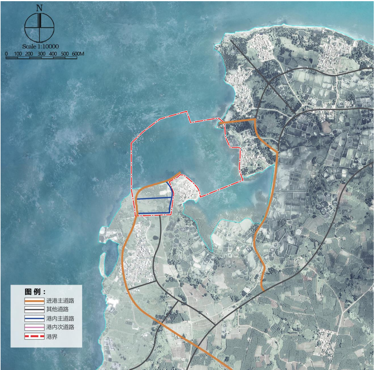
图 7.2-2 硇洲中心渔港（北港）交通规划图
