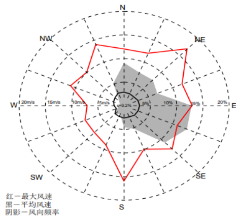
图 2.2-1 湛江风玫瑰图
