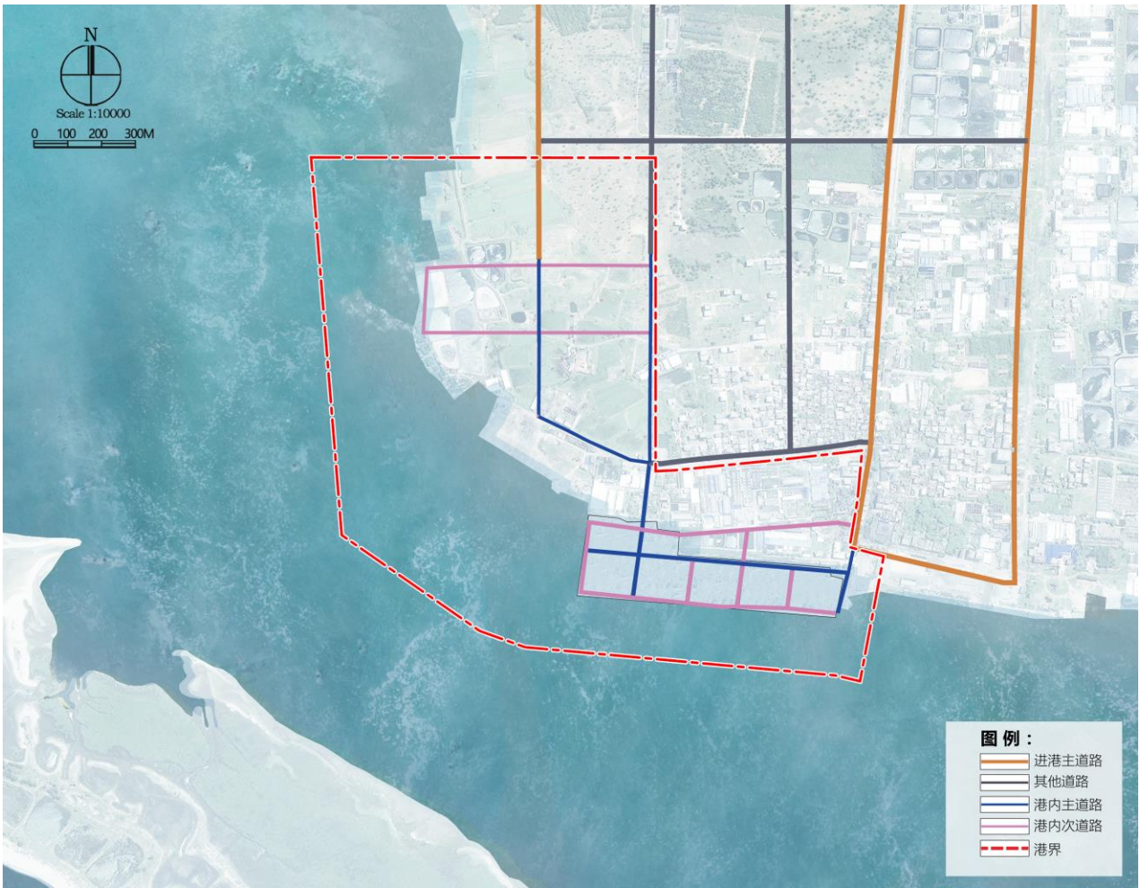
图 7.2-3 东南渔港交通规划图
