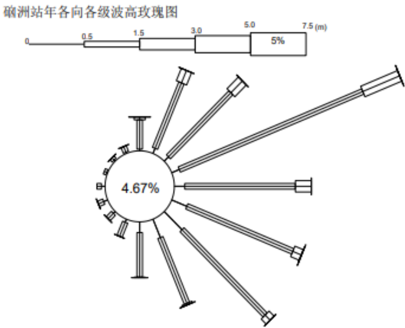
图 2-7 硇洲站各向波高玫瑰图
