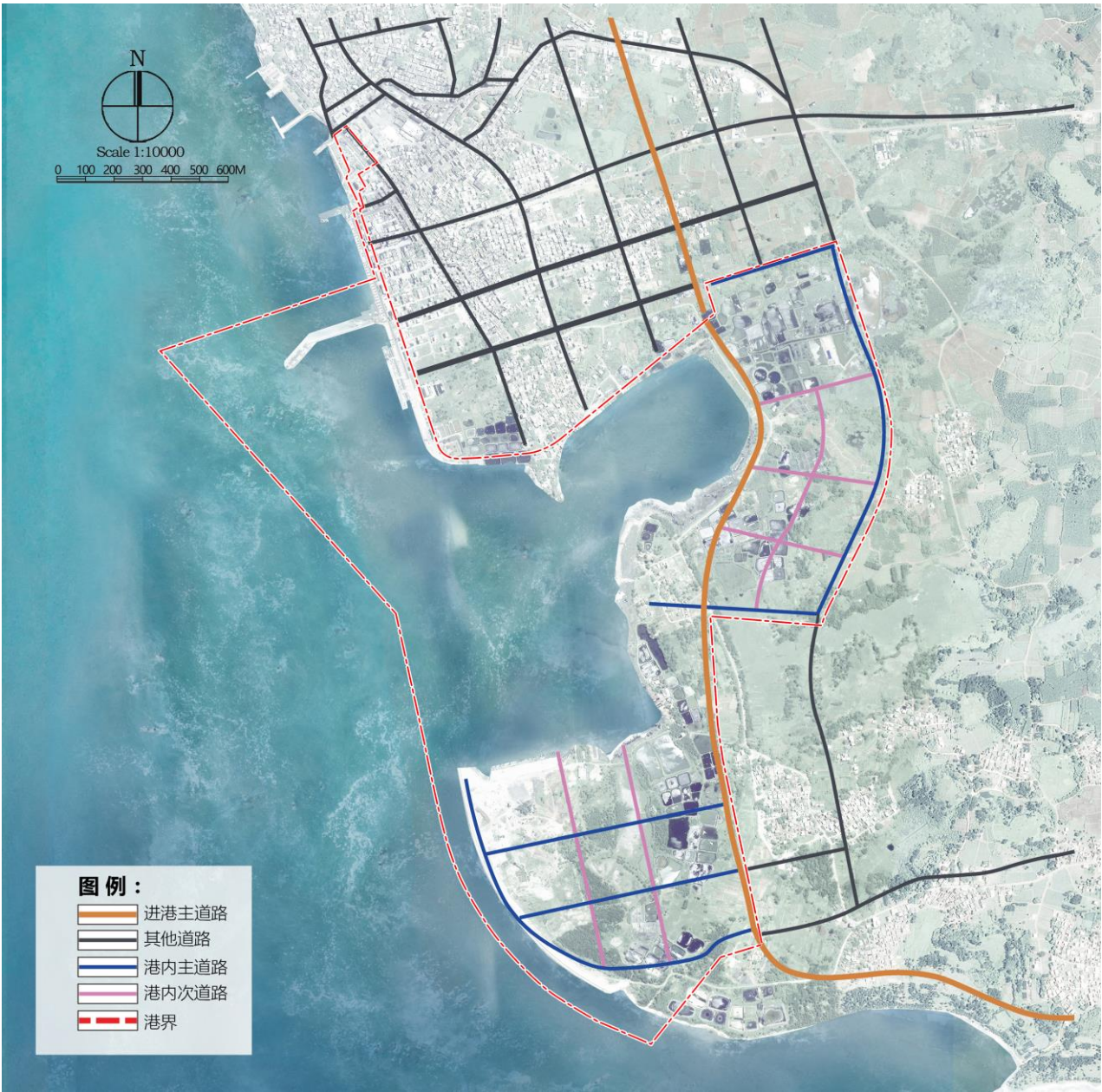
图 7.2-1 硇洲中心渔港交通规划图
