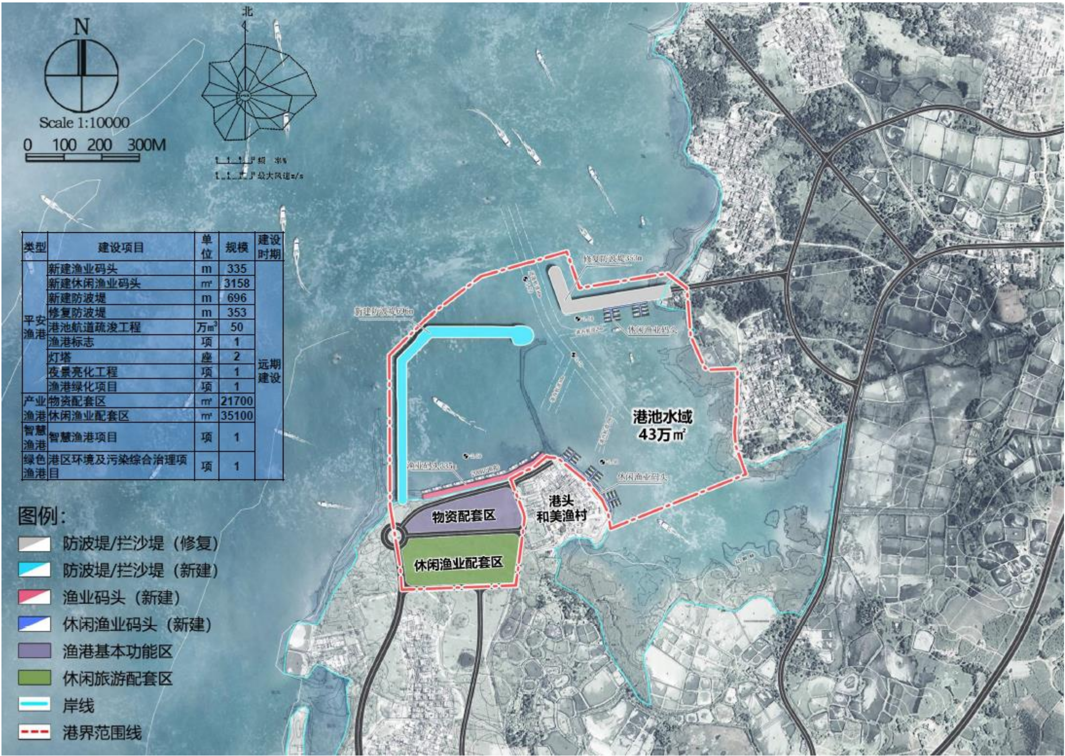
图 5.4-10 硇洲中心渔港（北港）功能布局图
