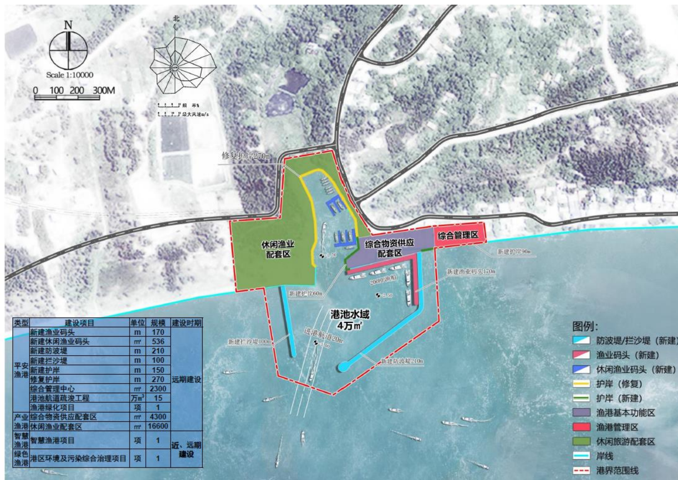
图 5.4-9 龙安渔港平面布局图
