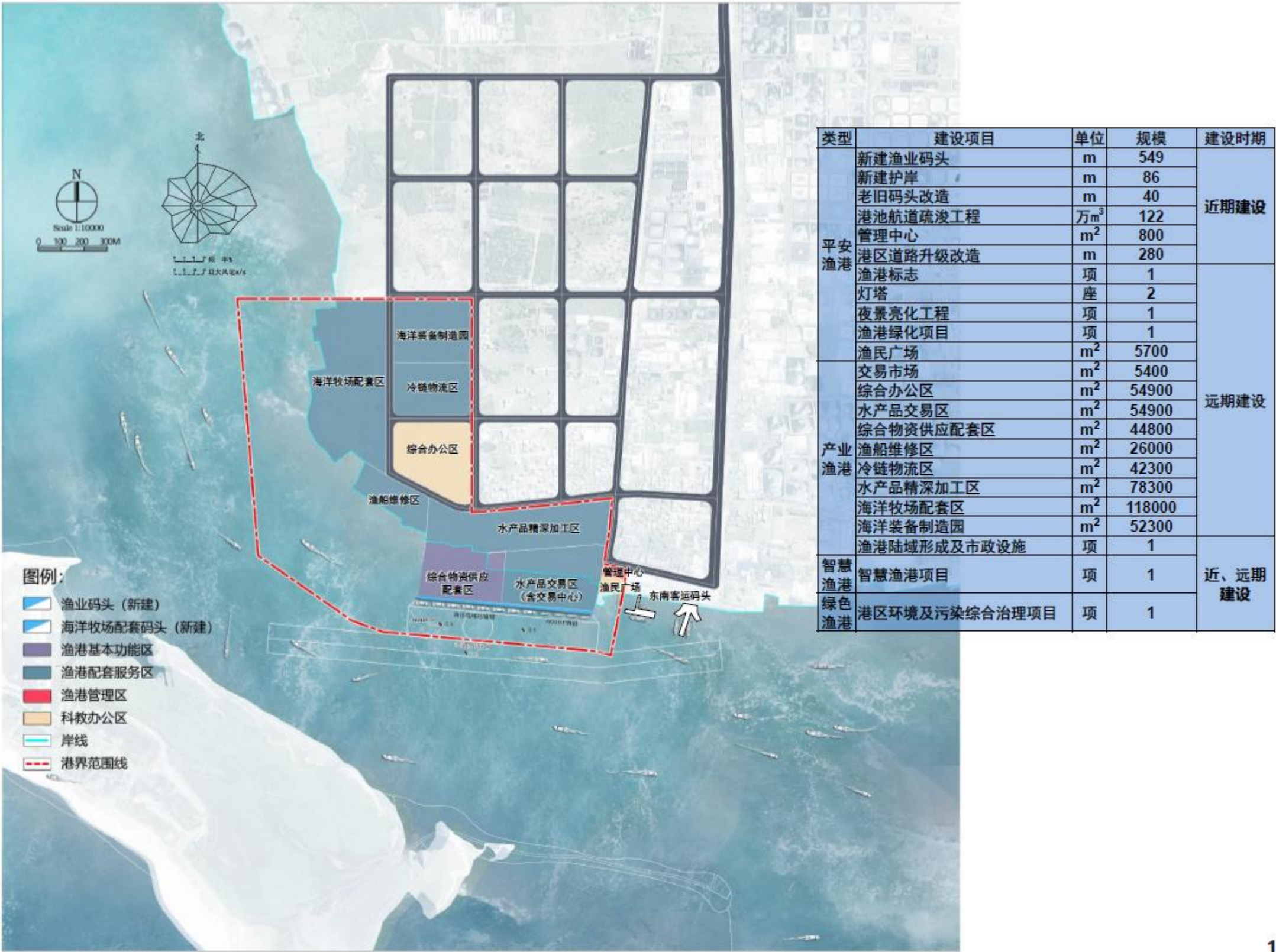
图 5.4-7 东南渔港功能布局图
